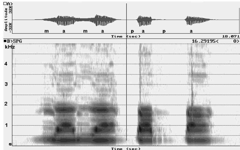
7. ábra Az előállított mama és a papa hangsorok szerkezete (oszcillogram és spektrogram)
